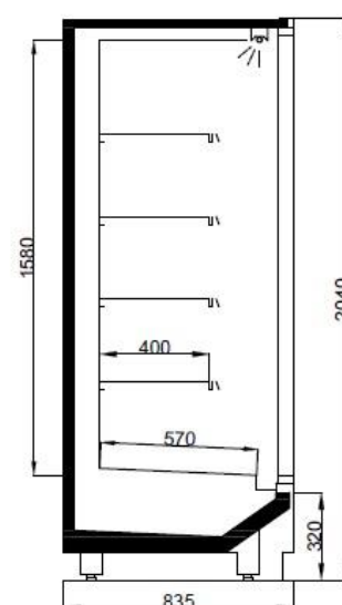
Πλάτος: 835mm
