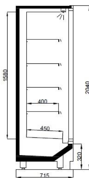
Πλάτος: 715mm
