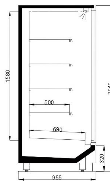
Πλάτος: 955mm
