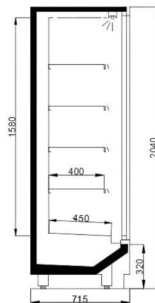
Πλάτος: 715mm
