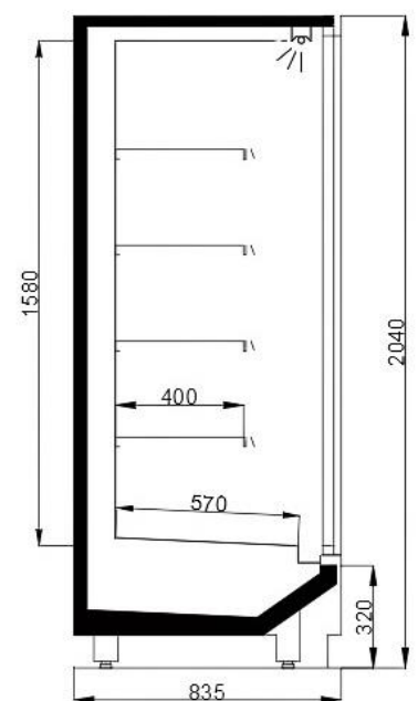
Πλάτος: 835mm
